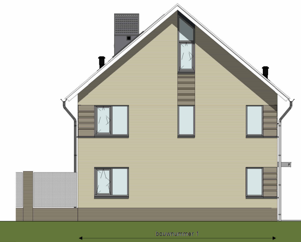
LINKERGEVEL
