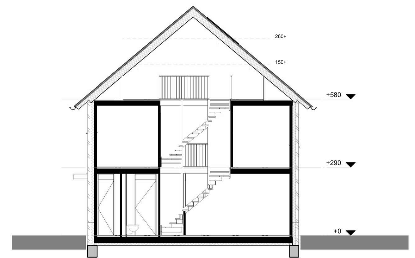
DWARSDOORSNEDE
