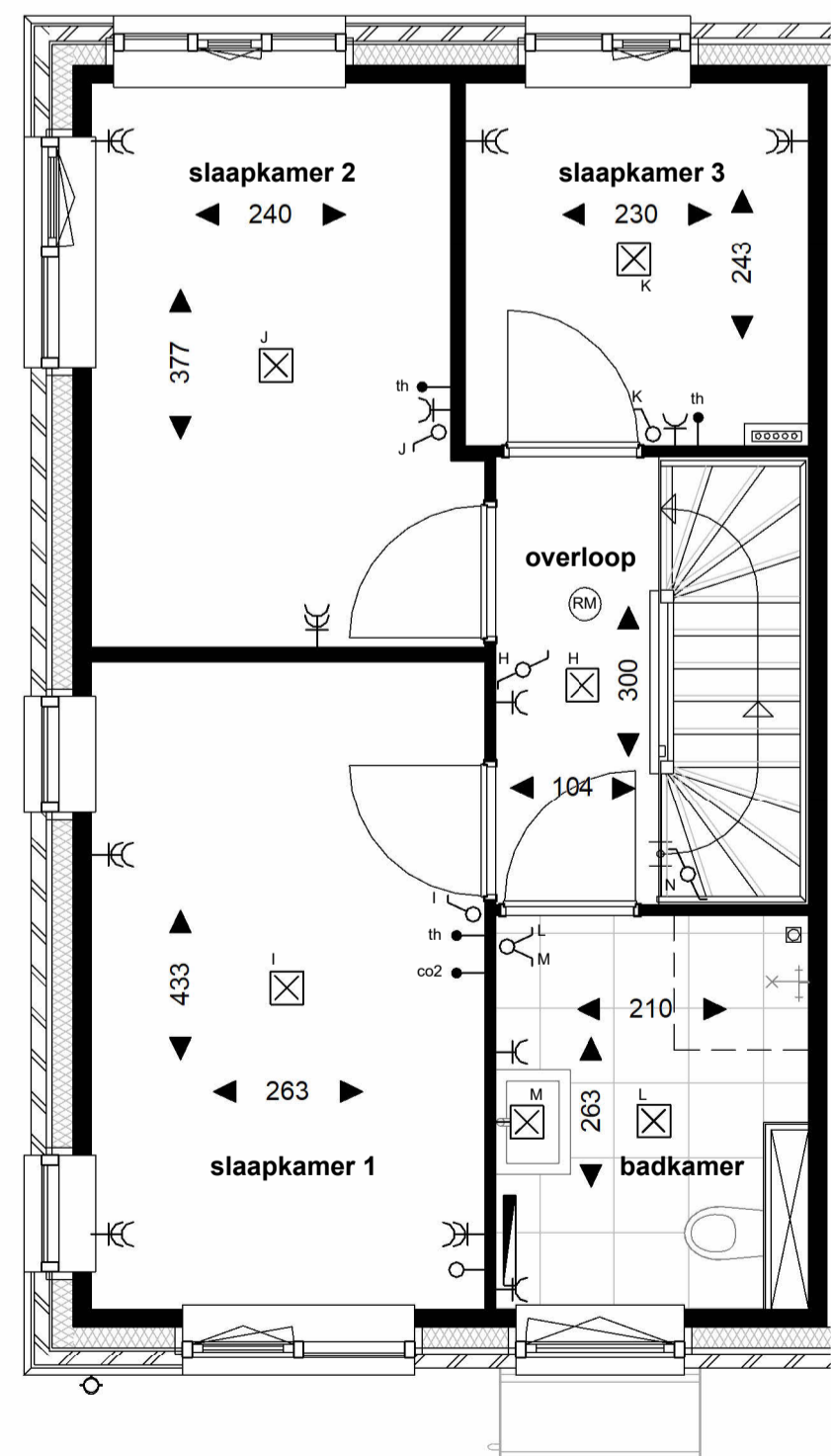
VERDIEPING 1
