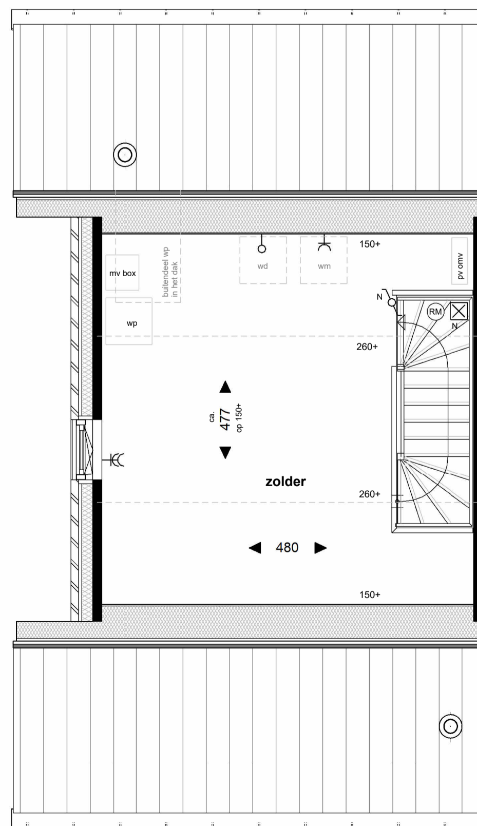
VERDIEPING 2
