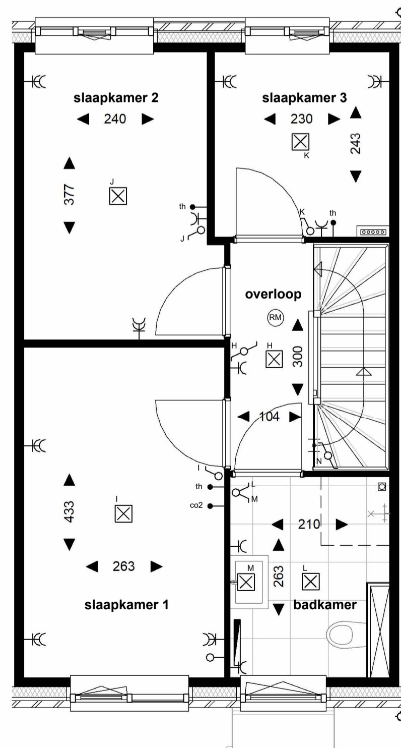
VERDIEPING
