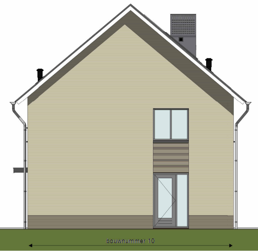
RECHTERGEVEL
