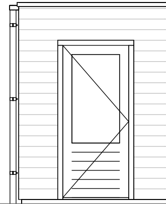
Rechtergevel
